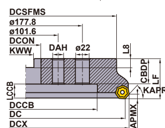
Fig.5 ø315
