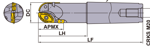
Kombischaft (Fig.7)
